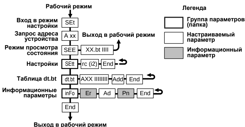
Рисунок 8 – Структура меню реле БПК при настройке с помощью показывающих и сигнализирующих приборов (например, МС-К-500-...)
