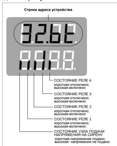
Рисунок 9 – Пример табло показывающего прибора при просмотре состояний реле БПК
